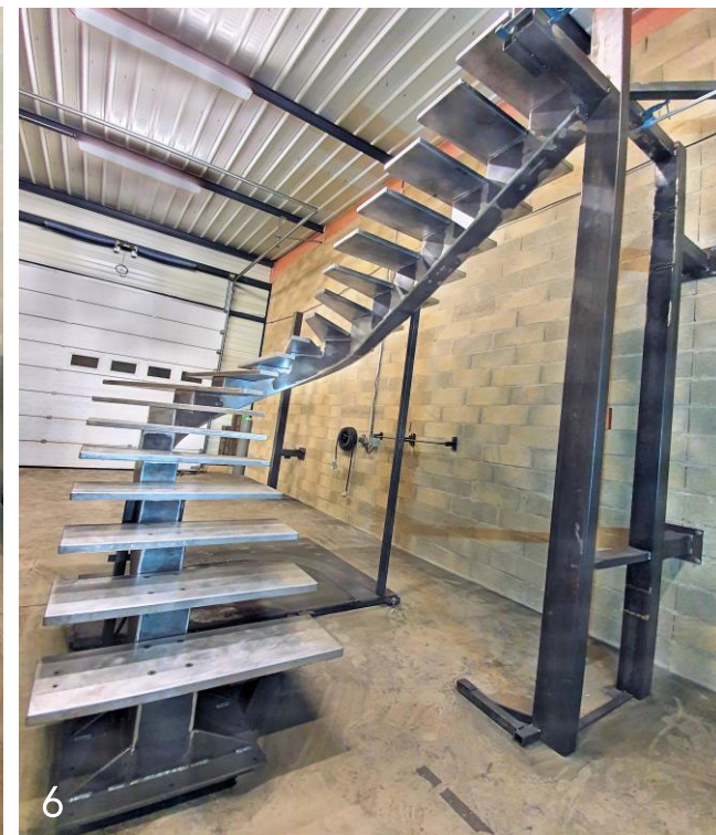
Exemple de réalisation 1 Conception | 2 Soudure | 3 Meulage | 4 Roulage | 5 Tôles découpées au laser | 6 Ouvrage complet
